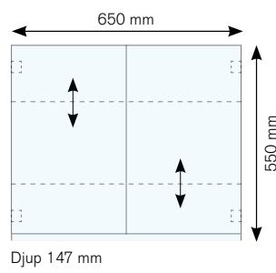
Djup 147 mm CRISTALLO 4 Ahlseil art.nr. 355608 RSK-nr. 8970079 Art nr. 2051004
