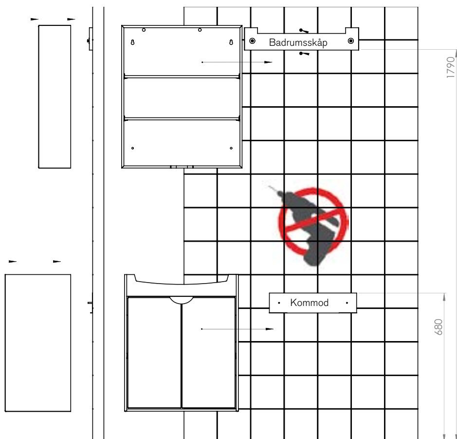
Borrfri upphängningsplåt för badrumsskåp och kommoder som limmas på kakel.
