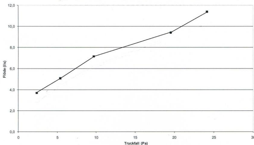
Diagram 1. Tryckfall-flöde över art nr: YSO 16012012
