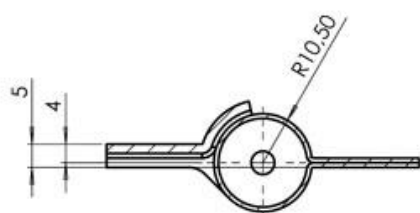
SCHNITT A-A
