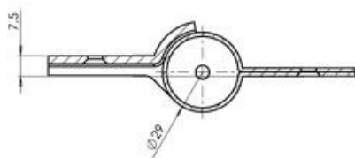
SCHNITT A-A
